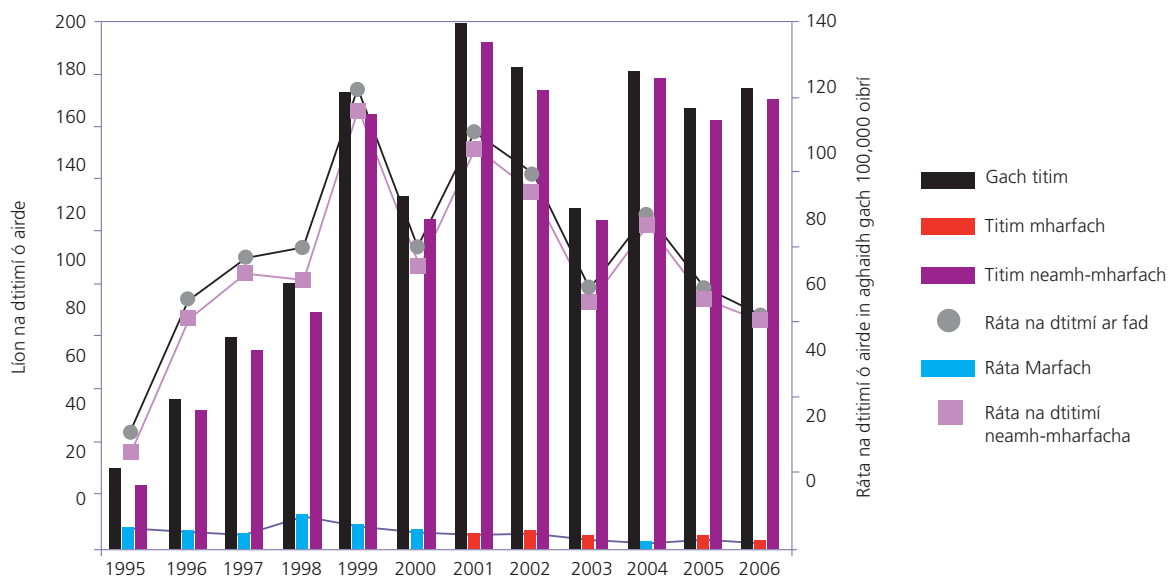
Fíor B.1: Timpistí a tuairiscíodh don HSA a bhain le titim ó airde de réir lín agus ráta in aghaidh gach 100,000 oibrí (HSA, 2007a, lch. 16)
