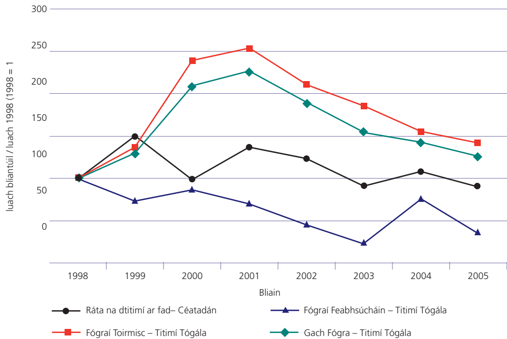
Fíor B.2: An t-athrú ar líon na bhfógraí a bhaineann le WAH a d'eisigh an HSA i dtionscal na tógála agus ráta na dtimpistí titime ó airde sa tionscal tógála a tuairiscíodh don HSA (1998 tógtha mar an mbonnlíne) (HSA, 2007a, lch. 46)
