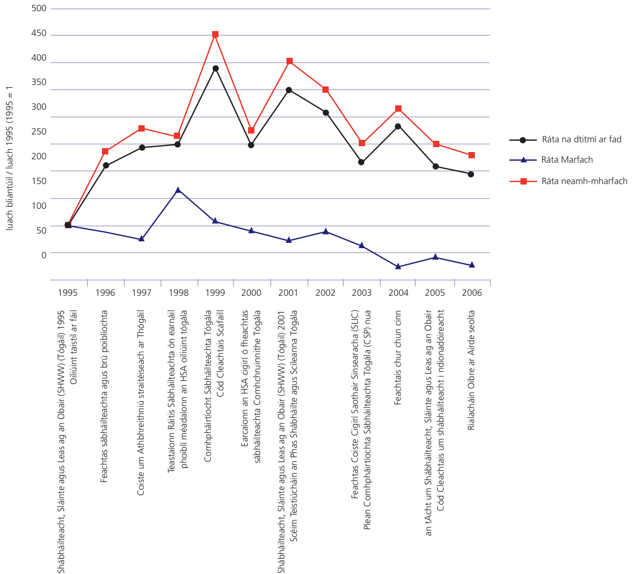
Fíor B.4: An t-athrú ar ráta na dtimpistí titime ó airde i dtionscal na tógála a tuairiscíodh don HSA (1995 tógtha mar an mbonnline) agus tionchar tionscnamh HSA (HSA, 2007a, lch. 43)
