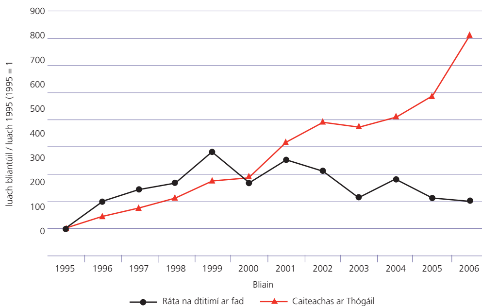
Fíor B.3: An t-athrú ar chaiteachas an HSA i dtionscal na tógála agus ráta na dtimpistí titime ó airde sa tionscal tógála a tuairiscíodh don HSA (1995 tógtha mar an mbonnlíne) (HSA, 2007a, lch. 47)
